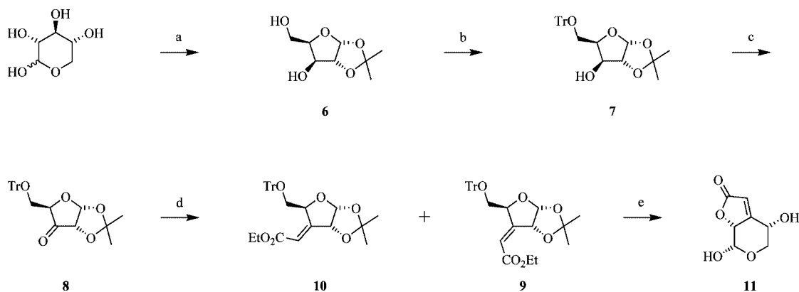
Scheme 3. (a) (i) \text{Me}_2\text{CO} , \text{H}_2\text{SO}_4 , (ii) \text{AcOH} , \text{H}_2\text{O} ; (b) \text{TrCl} , \text{Et}_3\text{N} , \text{CH}_2\text{Cl}_2 ; (c) \text{Ac}_2\text{O} , \text{Me}_2\text{SO} ; (d) \text{NaH} , (\text{EtO})_2\text{POCH}_2\text{CO}_2\text{Et} , THF ( 10 / 9 , 1:19), 5% and 74% from 7 , respectively; (e) \text{CF}_3\text{CO}_2\text{H} , \text{H}_2\text{O} , 83%.
